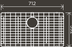
Lavello Protection Grid for MKSP-S760440
