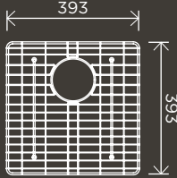
Lavello Protection Grid for MKSP-S450450
