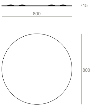
SPT80 Specchio rotondo con illuminazione led perimetrale Round mirror with led sorround backlight Ø80
