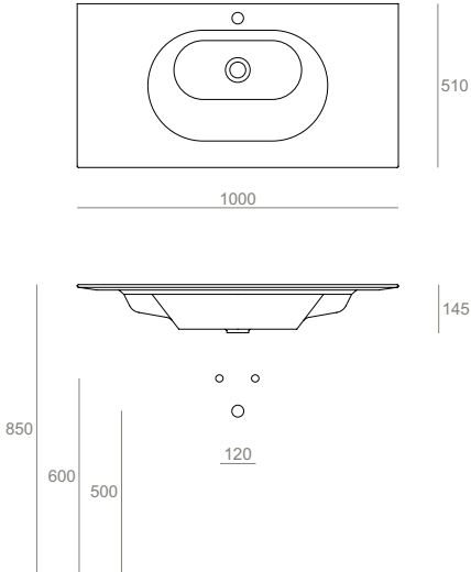
WA100 Piano lavabo 100 sospeso monoforo con bacino ovale - H. top 0,8 Single hole wall-hung top 100 with oval basin - Top thk 0,8 100.51.14,5
