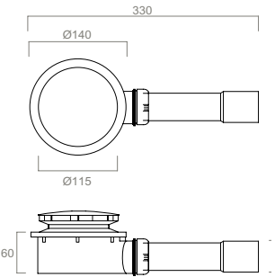
PH6 Piletta per piatto doccia con tappo in plastica cromata Shower waste with chromed plastic plug
