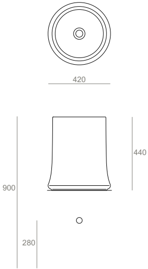
SH10 Lavabo Ø42 tondo da appoggio Round countertop washbasin Ø42 Ø42.44
