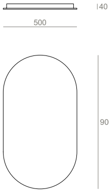
SP050 Specchio ovale con illuminazione led perimetrale Oval mirror with led sorround backlight 50.90
