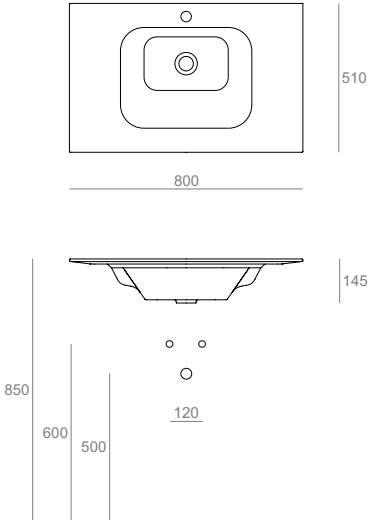
WA80 Piano lavabo 80 sospeso monoforo con bacino rettangolare - H. top 0,8 Single hole wall-hung top 80 with rectangular basin - Top thk 0,8 80.51.14,5
