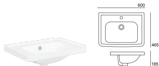
Lavatório . Lavabo . Washbasin 16381XX2C
