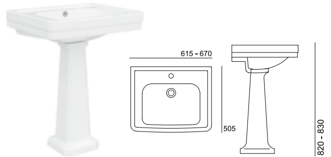
Lavatório . Lavabo . Washbasin
